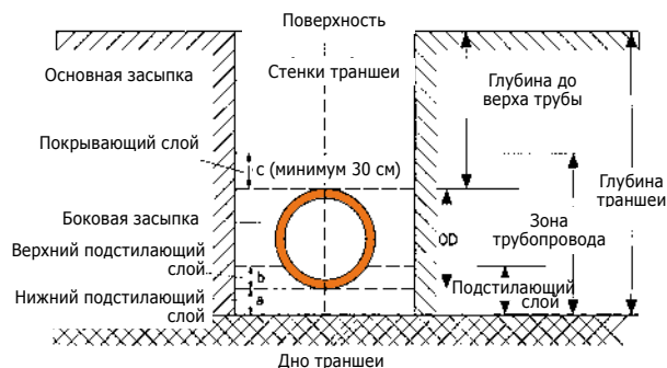
Рис. 3 Устройство траншеи
